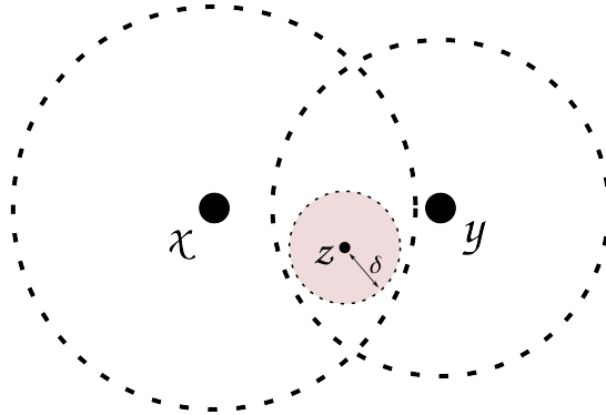
Figura 1.4: Para cada ponto z da interseção B_{\varepsilon_1}(x) \cap B_{\varepsilon_2}(y) , temos uma “bolinha” centrada em z e toda contida na interseção.
